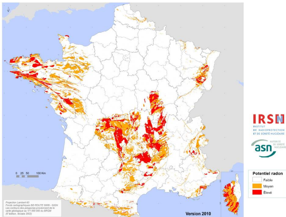
POTENTIEL RADON DES FORMATIONS GEOLOGIQUES A L'ECHELLE 1 : 1 000 000 (VERSION 2010)
