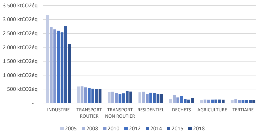
EVOLUTION DES EMISSIONS DE GAZ A EFFET DE SERRE ENTRE 2005 ET 2018
